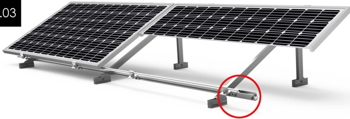
Kit 1 - Fijar las uniones del perfil guía inferior mediante los tornillos de martillo (2 a cada lado de la unión) Repetir en perfil guía superior.
