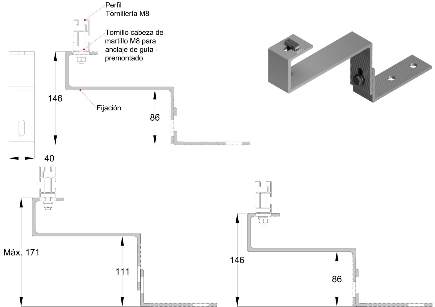
Distancias mínima y máxima de regulación en altura, distancias de anclajes
