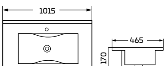
Lavabo 100
