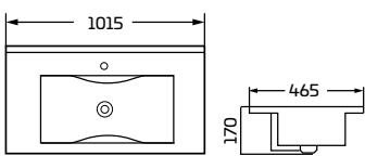
Lavabo 100
